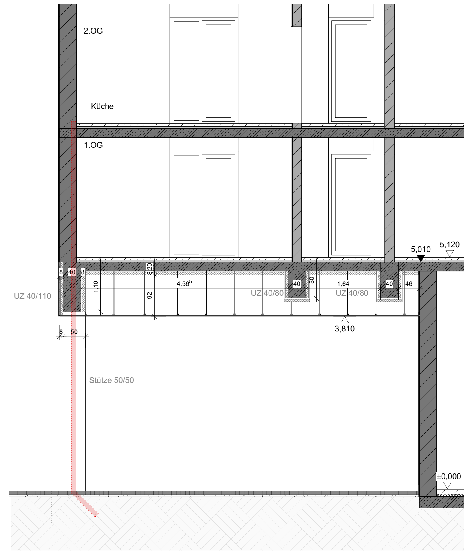
Schnitt D-08
