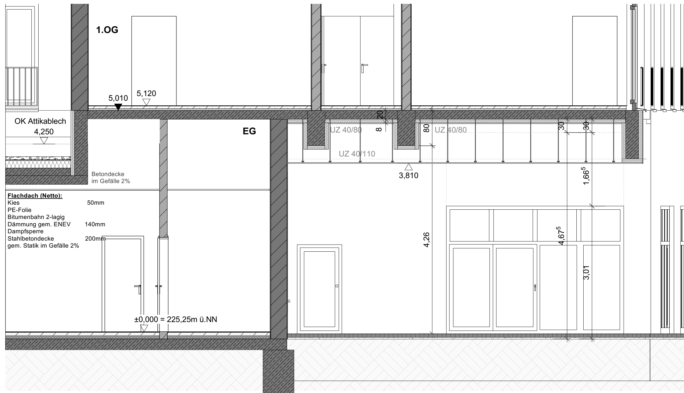
Schnitt D-01
